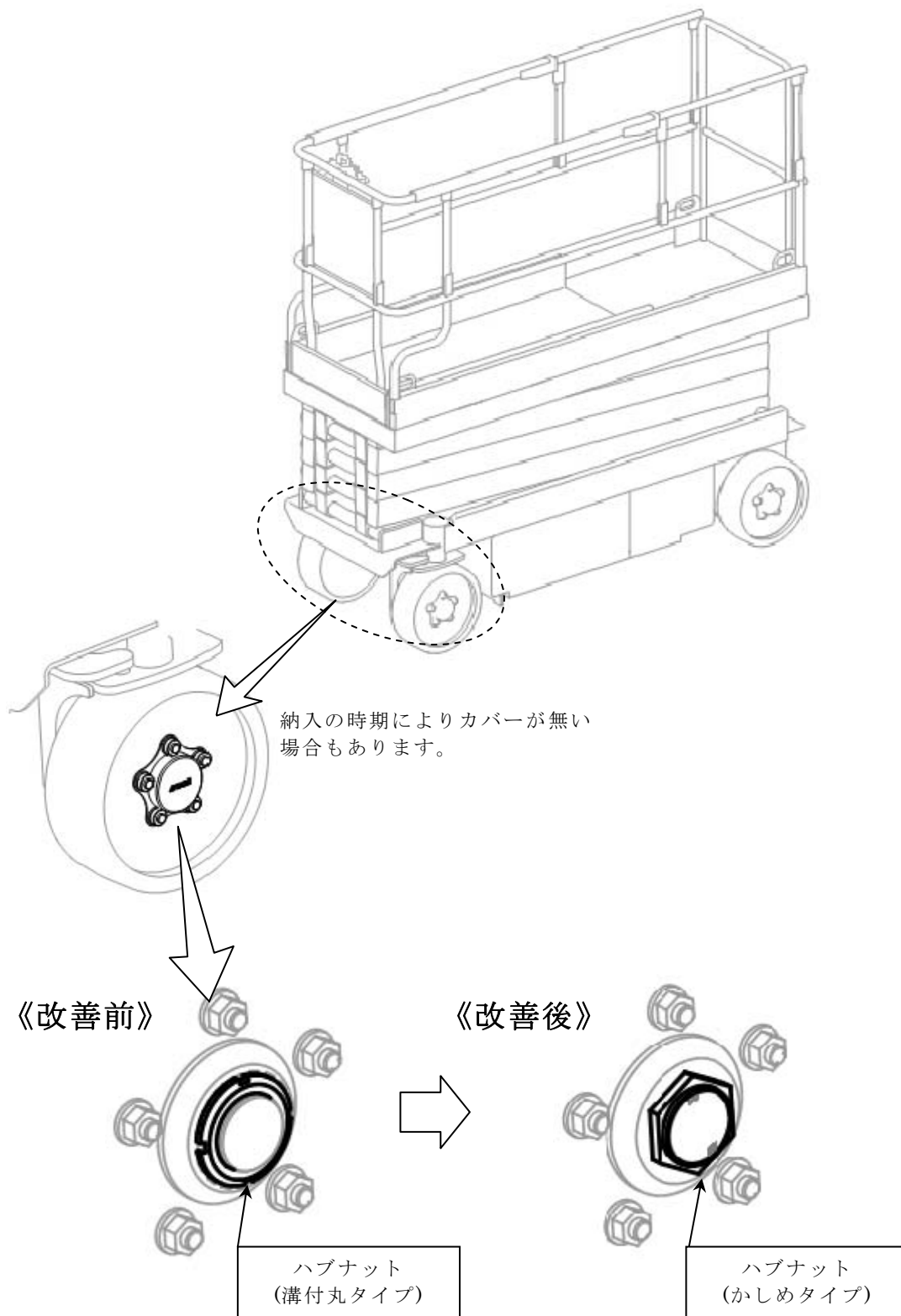
図1 改善箇所説明図(図は SV06DNS)
